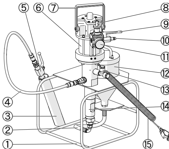
Fig. 5: HD 1
